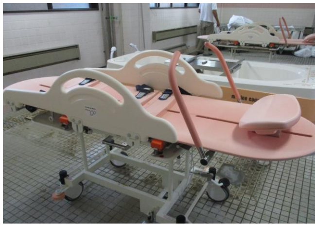
フラット担架（上部分）・コンパクトストレッチャー（下部分）
